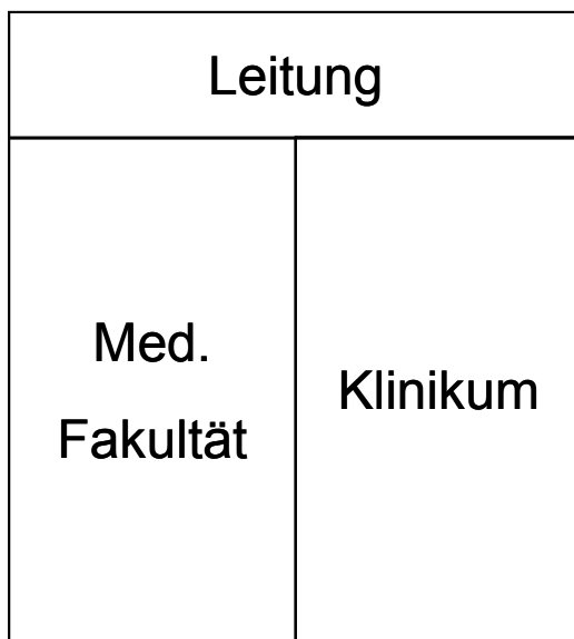
Abbildung 2: Integrationsmodell
